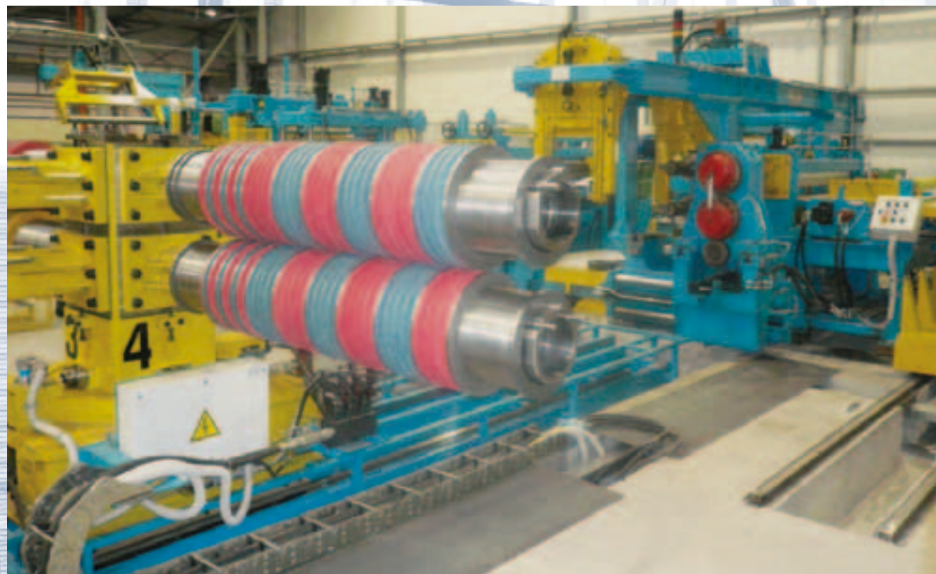
▲ Linea di taglio longitudinale 1600 x 3, 5 con giostra automatica cambio lame, installata in Polonia
